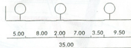
SECCION 3 ENTRE EDIFICIO ENET No 10 Y AV. CASEROS.
