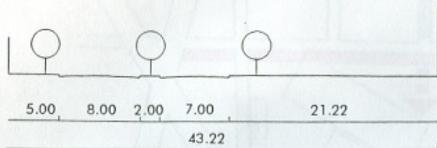
SECCION 1 AV. AVELLANEDA Y J. CANNING
